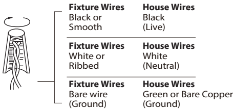
Fig. 3 Wiring
