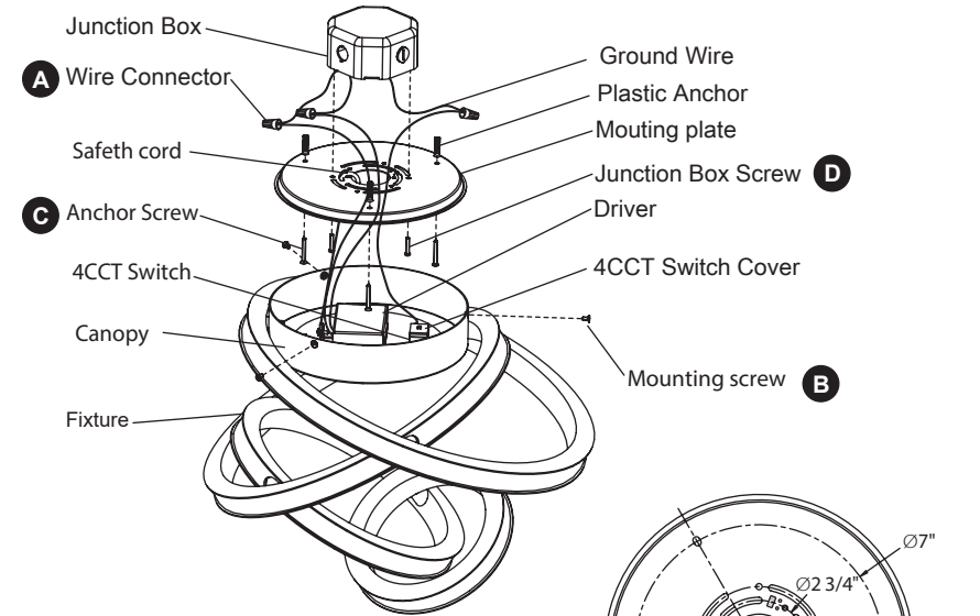
Fig. 2 Wiring
